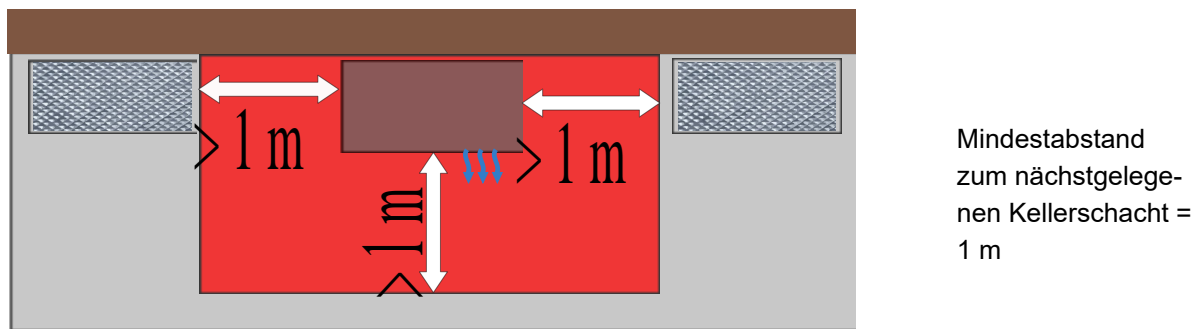
Abbildung 8: Draufsicht der Aufstellung an einer geschlossenen Wand
