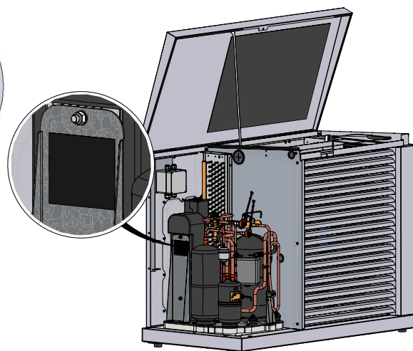
Abbildung 2: Typenschild Innen
