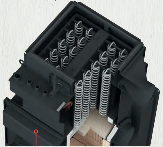
HKD 2.2 SK mit integrierter Reinigungsmechanik
