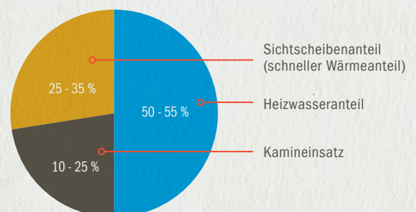
Aufteilung der nutzbaren Wärmemenge
