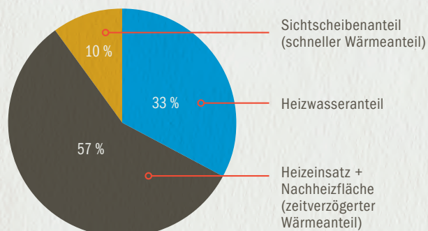
Aufteilung der nutzbaren Wärmemenge
