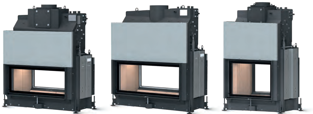
Architektur-Kamin Tunnel 38/86 mit Kesselaufsatz
