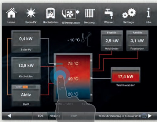
Touchdisplay mit Home-Ansicht der Heizzentrale BHZ
