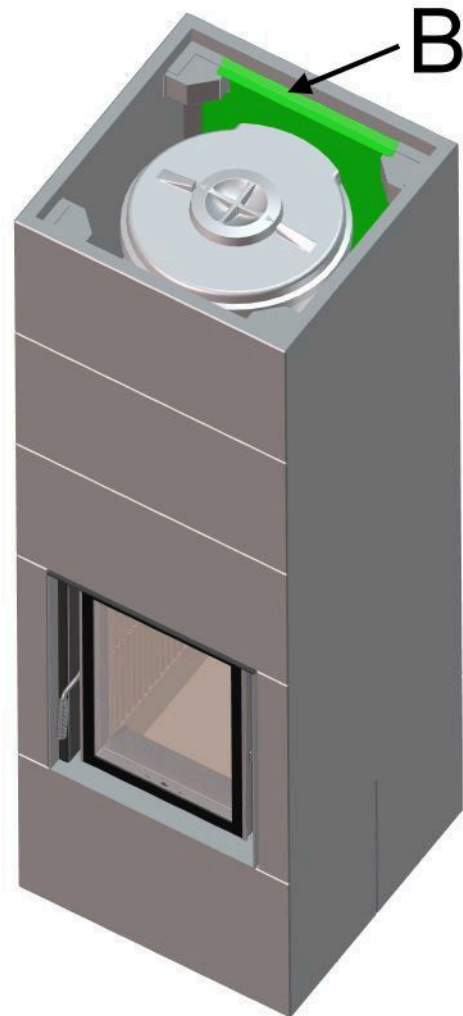
Abb. 6: Einbaulage der Hitzeschutzbleche (B)
